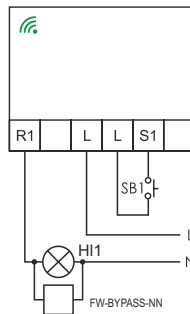
Схема подключения FW-R1P-NN с применением FW-BYPASS-NN
